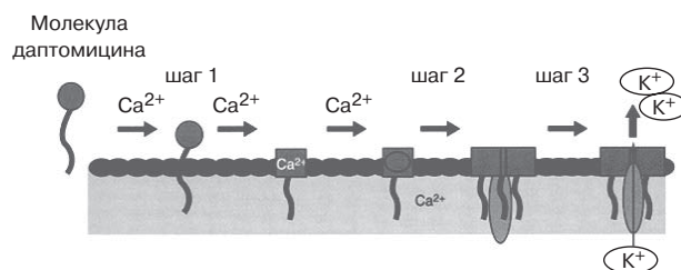
Рис. 3. Механизм действия даптомицина [10]. шаг 1 – кальций-зависимое связывание и встраивание липофильного «хвоста» в цитоплазматическую мембрану; шаг 2 – олигомеризация и формирование ионных каналов; шаг 3 – выход ионов калия из клетки, приводящий к деполяризации мембраны и смерти микробной клетки.
